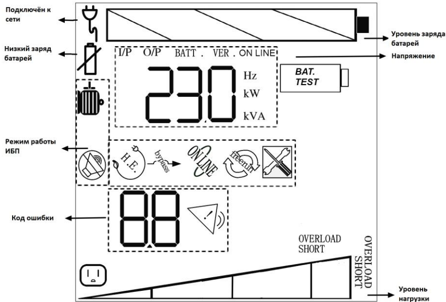
Рис. 7. ЖК-дисплей
