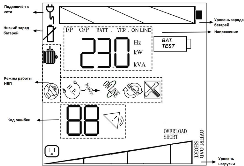
Рис. 6. ЖК-дисплей
