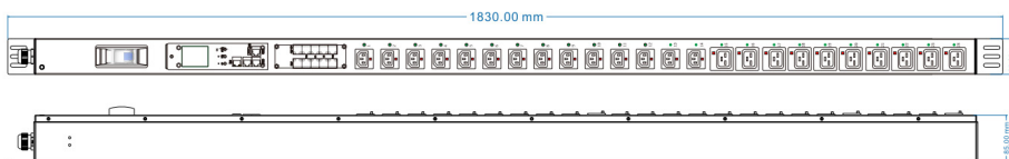
Модель PDU-32AVMS24-14C3-10C9-1P блок распределения питания с модулем «Smart Intelligent PDU», 1 фаза 24 розеток
