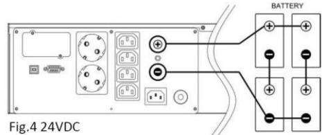
Рис.4 24 В пост. тока
